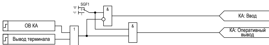
Рисунок 2.28 – Логика управления режимами функционального блока «КА»
