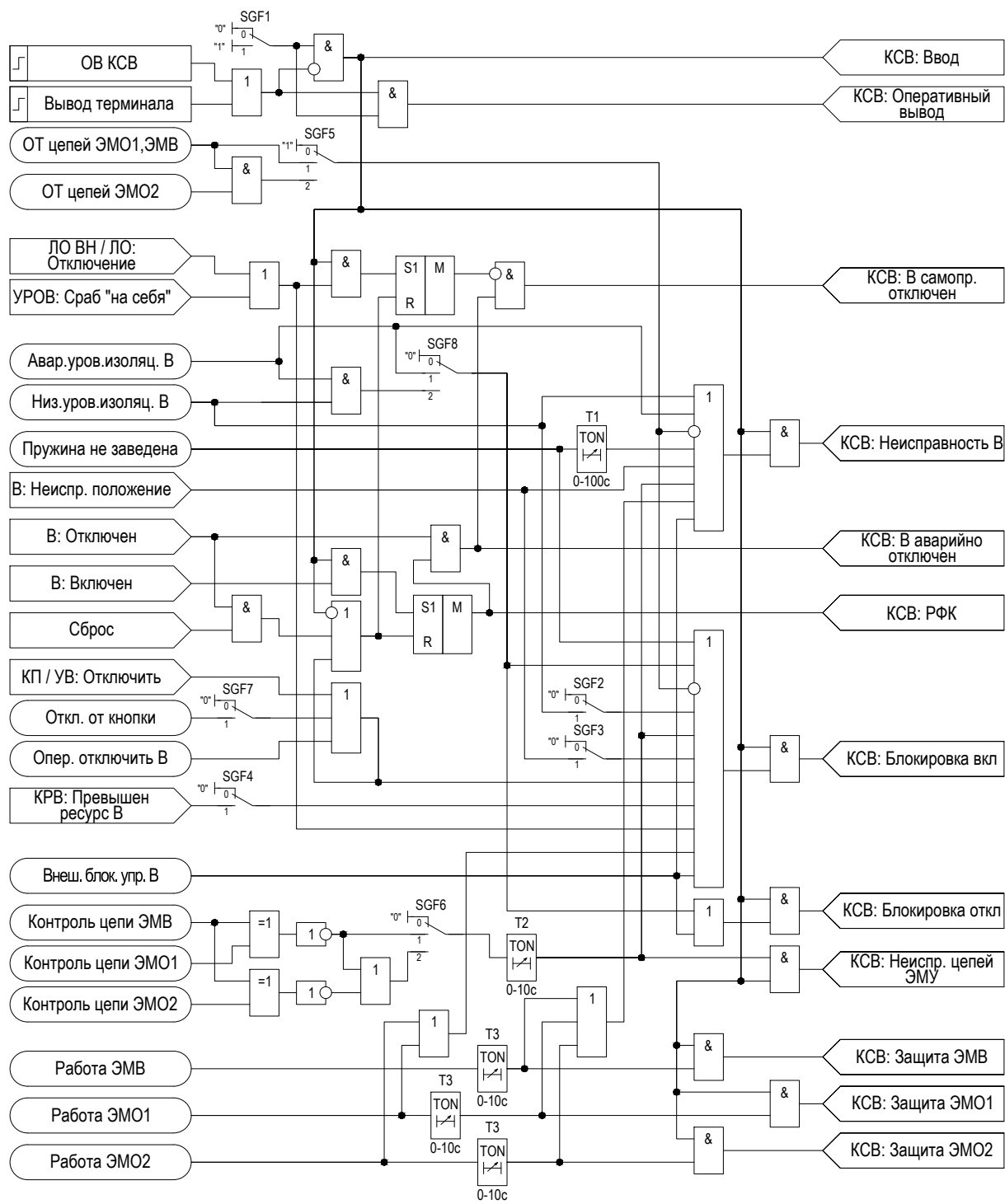
Рисунок 2.24 – Функциональная схема «КСВ»
